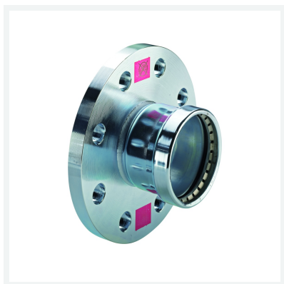
Prestabo XL karimás átmeneti idom SC-Contur-ral (biztonsági kontúr) modellszám 1159XL cikkszám 598 211
